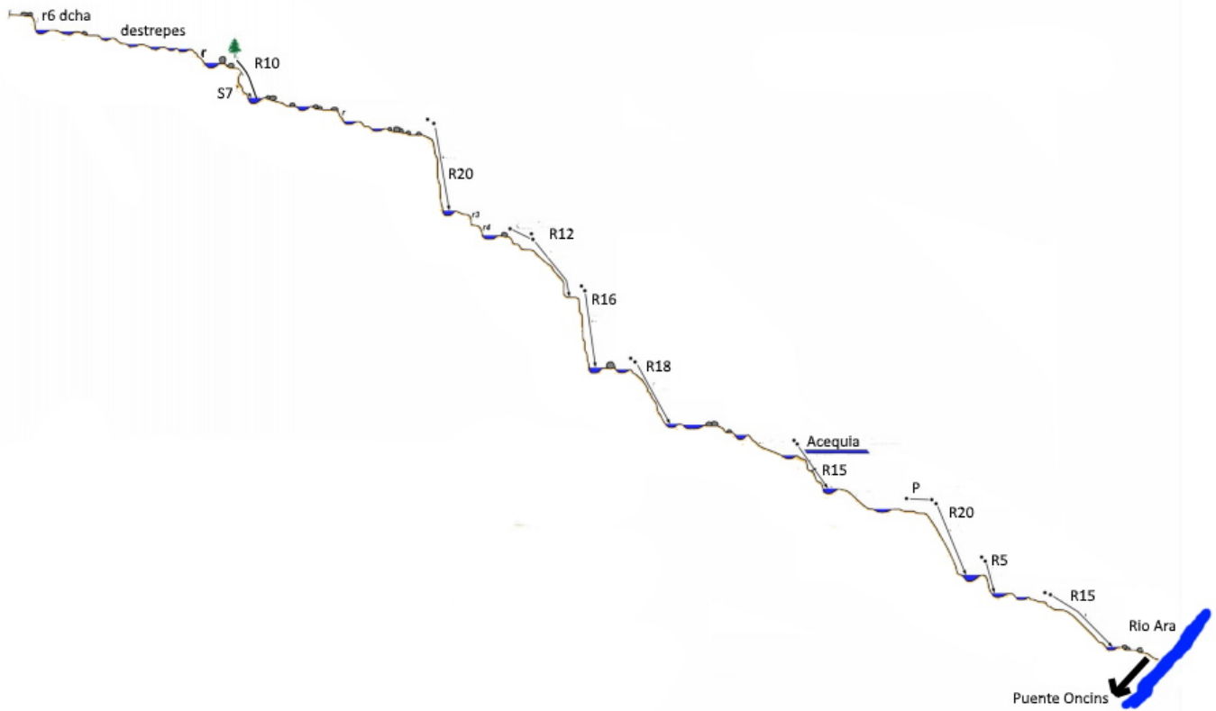
Imagen: Topografía barranco de Otañal
